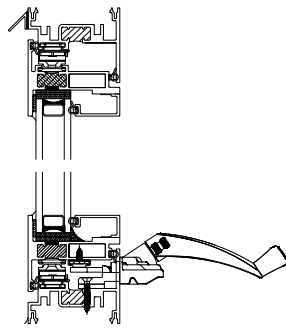
G2 Casement
