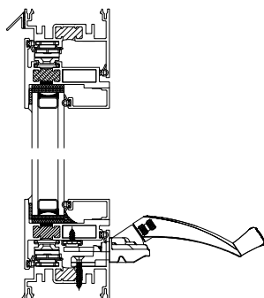
G2 HP Tilt Turn
