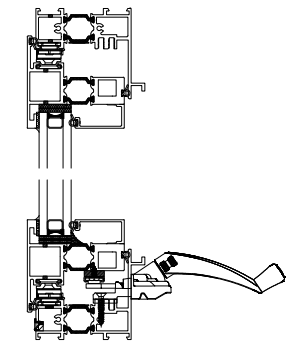
G3 Casement
